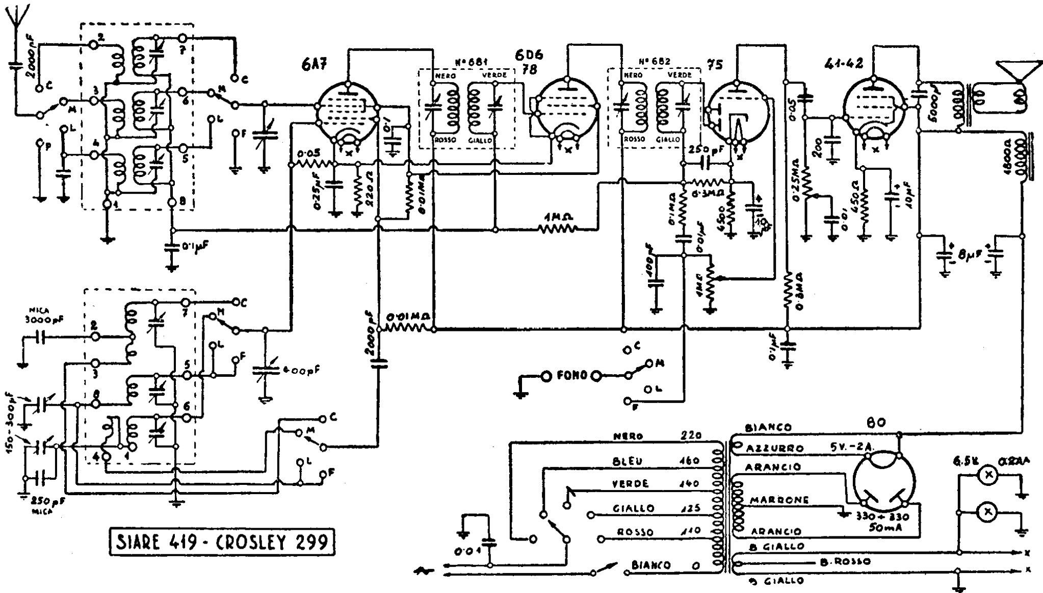
RADIO SIARE — Modelli « Siare 419 » e « Crosley 299 » · Produzione 1937 Media frequenza: 468 kHz.
